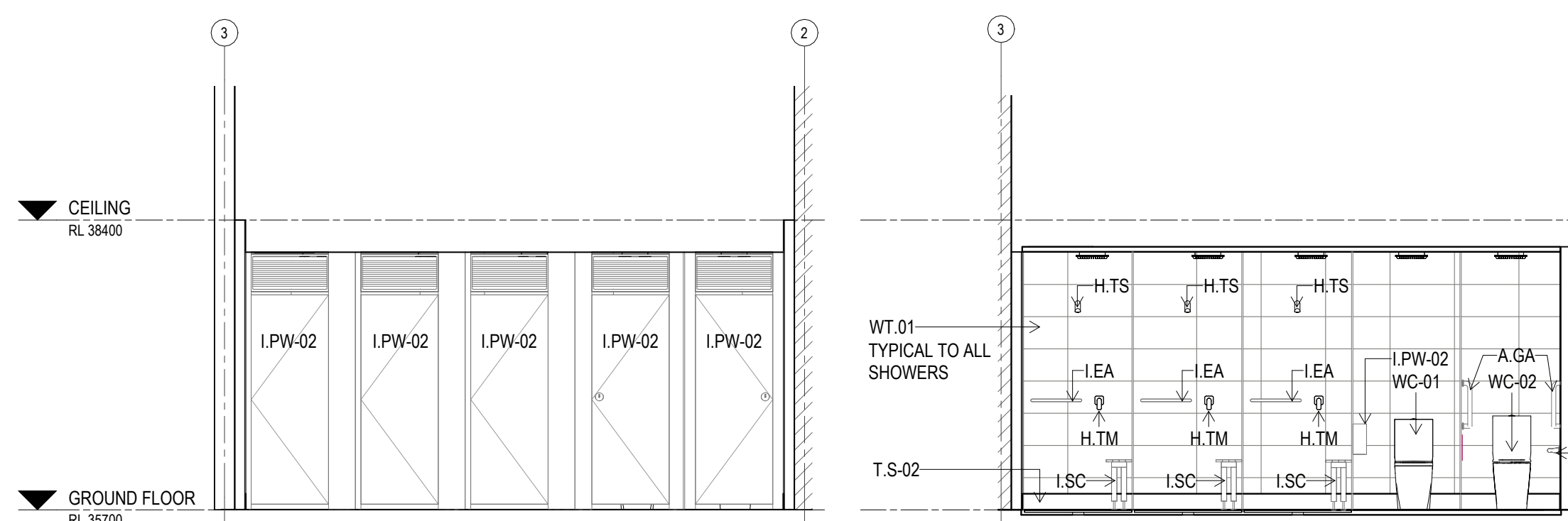
E ELEVATION CHANGE ROOM 1 Scale: 1 : 50
